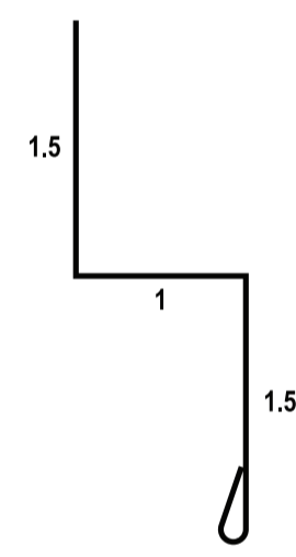
15. DOUBLE ANGLE
