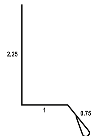
16. DRIP CAP
